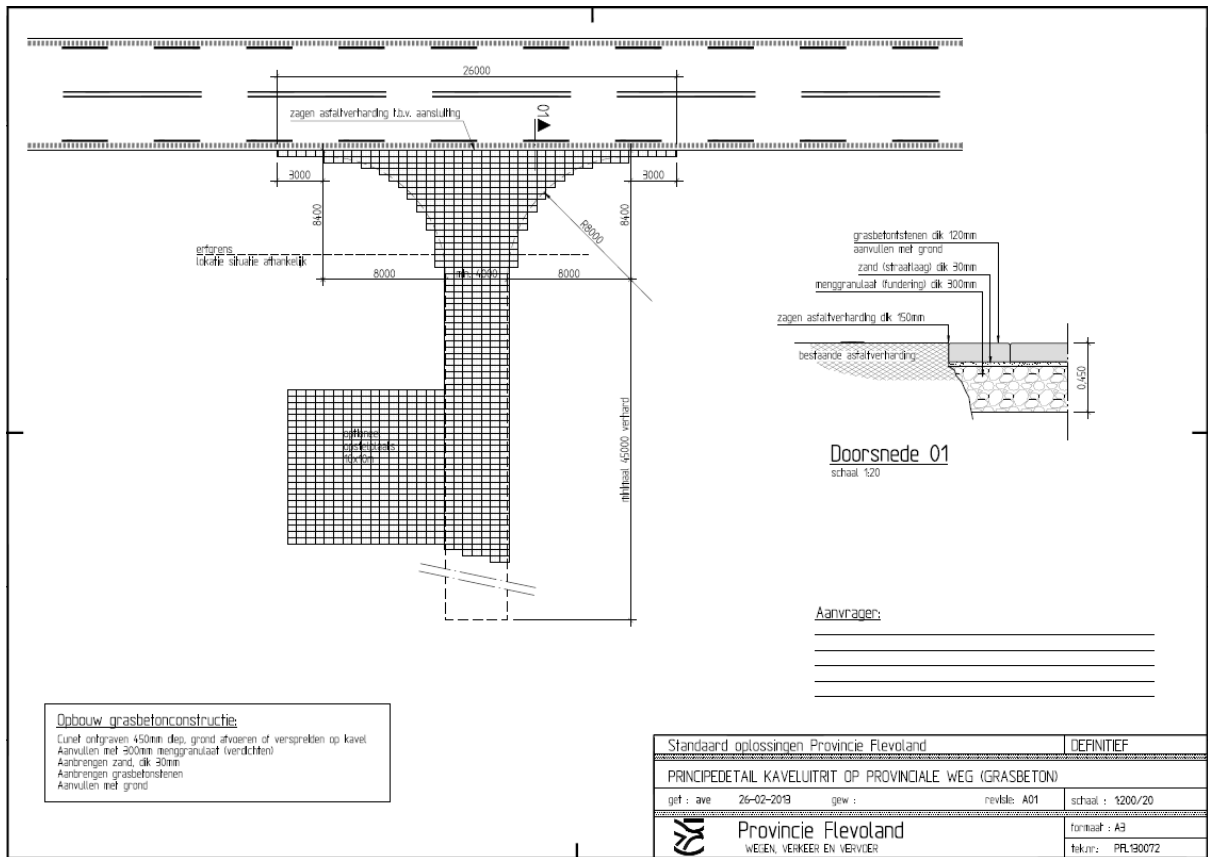
Situatietekening 2.5. Principedetail kaveluitrit op provinciale weg (grasbeton)
