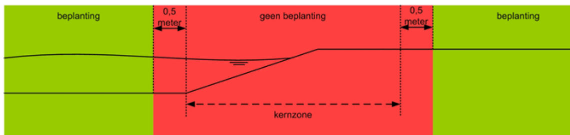
Figuur AR1.5: beplanting kadastrale erfafscheiding verheelde en aangeheelde waterkering
