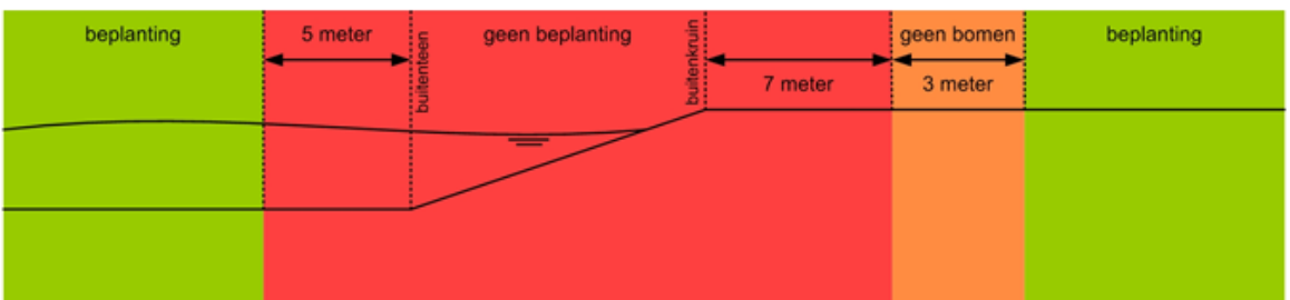
Figuur AR1.4: beplanting verheelde en aangeheelde waterkering
